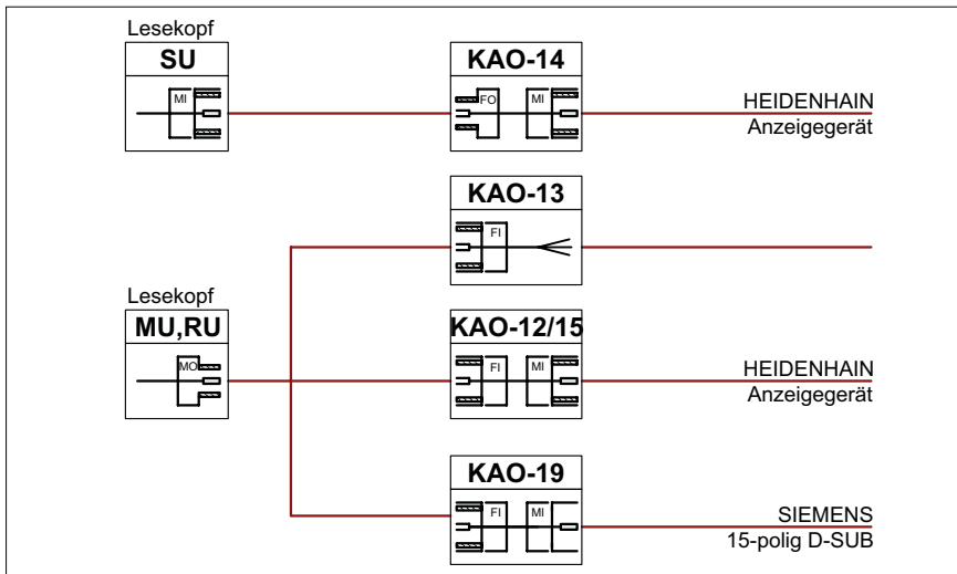
Kabel für analoge Leseköpfe
