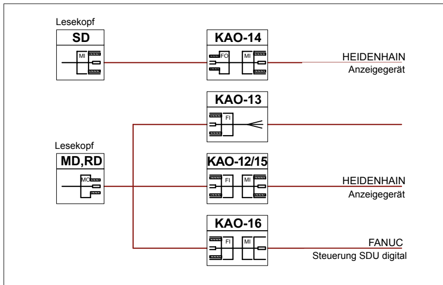
Kabel für digitale Leseköpfe
